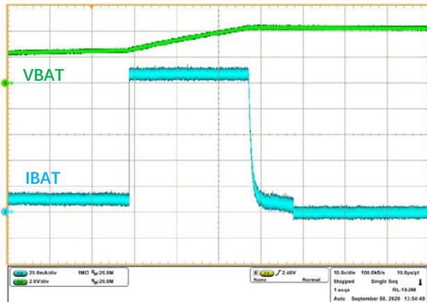
充电波形
