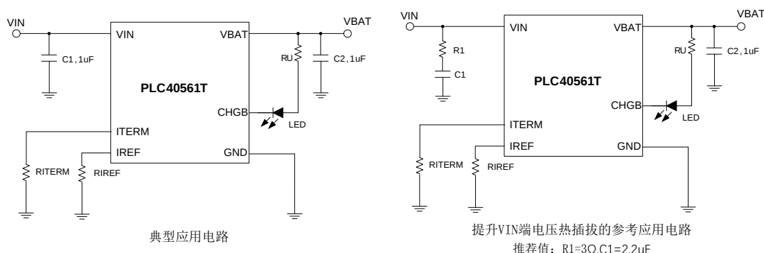
图 1 应用电路
